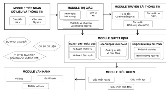
Hình 1: Cấu trúc điều khiển trong xe tự hành
