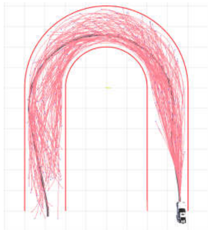
Hình 4: Thiết lập đường đi bằng Cây RRT [37]
