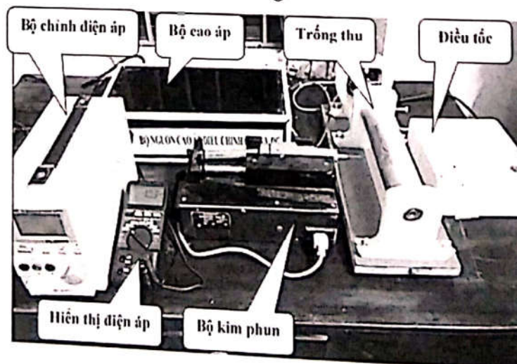
Hình 1. Thiết bị quay điện E-HUSC-02
