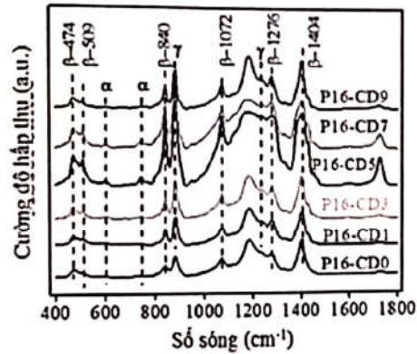
Hình 5. Phổ FTIR của màng PVDF với các nồng độ CDs khác nhau
