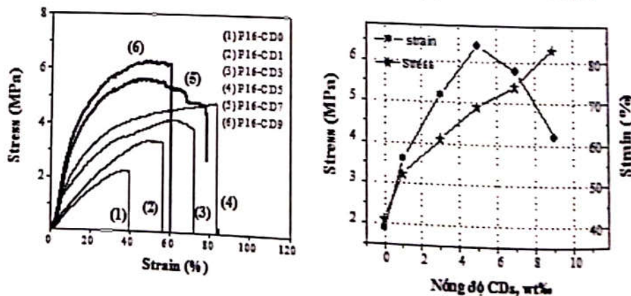
Hình 8. Ứng suất lực và độ dãn tương đối của vật liệu PVDF/CDs
