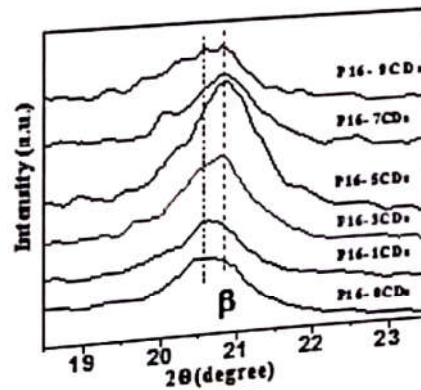
Hình 6. Phổ XRD của màng PVDF 16%kl với các tỉ lệ pha tạp CDs khác nhau
