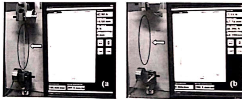
Hình 7. Thiết bị kiểm tra độ bền màng ghi lại kết quả cặp dữ liệu: giá trị lực kéo F(N) , độ dãn dài \Delta l(mm) của màng PVDF/CDs, trước khi đứt (a) và sau khi đứt (b)
