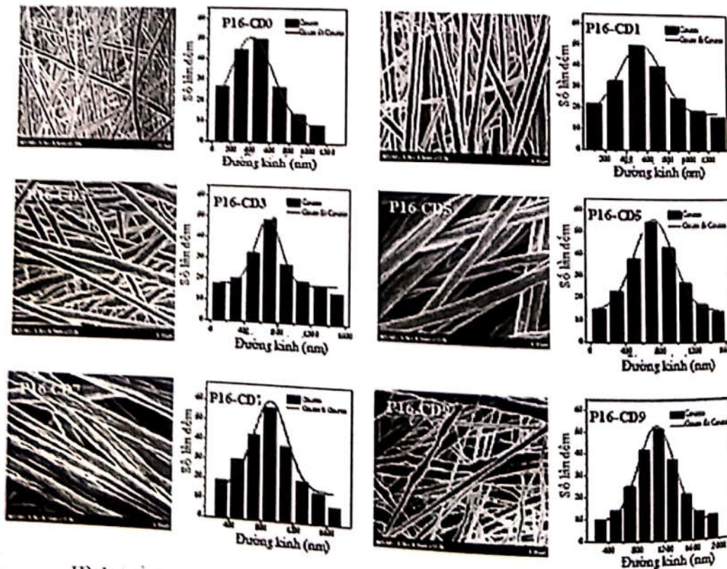
Hình 4. Ảnh SEM và đường phân bố kích thước sợi của màng PVDF
