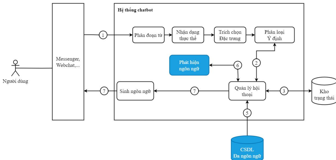
Hình 1. Mô hình chatbot đa ngôn ngữ được phát triển dựa trên kiến trúc đơn ngôn ngữ của RASA
