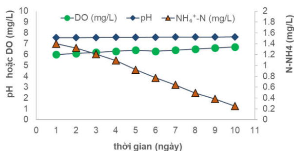
Hình 2. Biến động các thông số \text{NH}_4^+\text{-N} , DO, và pH ở pha khởi động (10 ngày)
